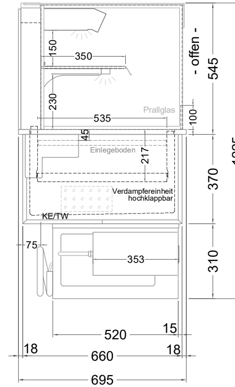
(Seitenansicht)
