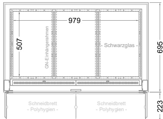
(Grundriss)
