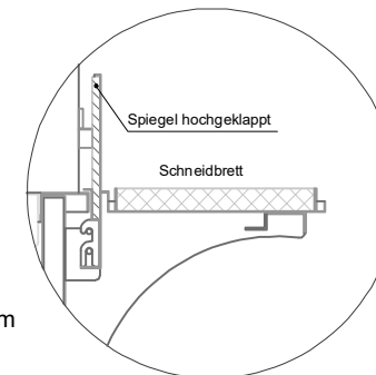
(Detail Spiegelsystem)
