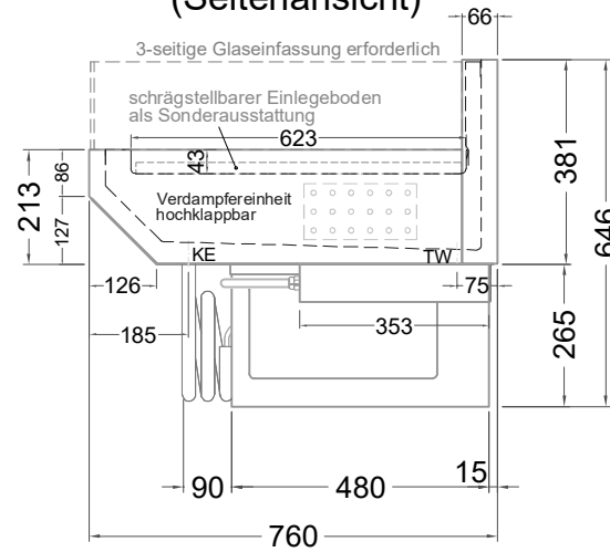
(Seitenansicht)
