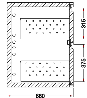
Schnitt L1
