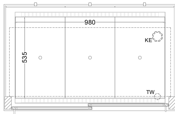
(Grundriss)
