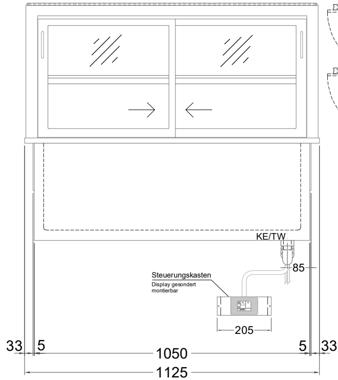
(Bedienseite)
