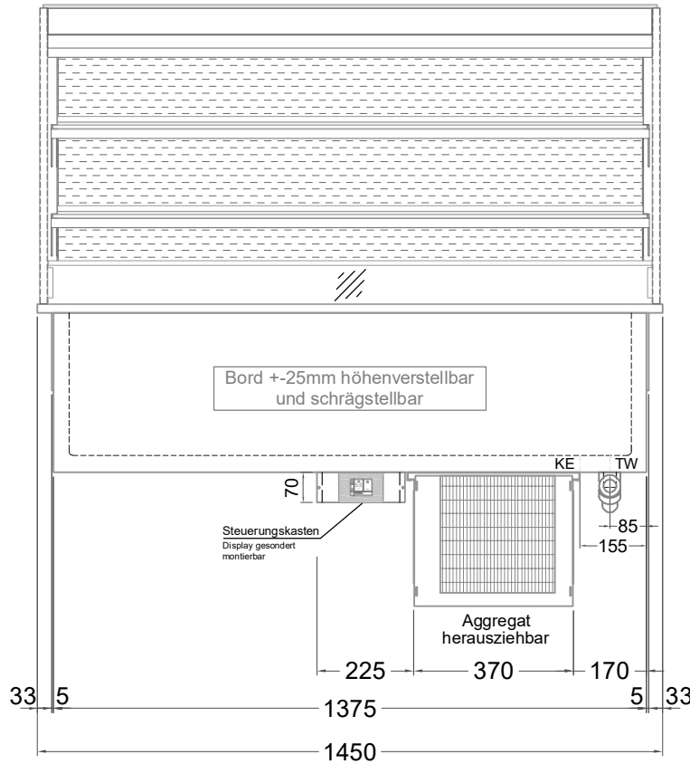
(Grundriss)
