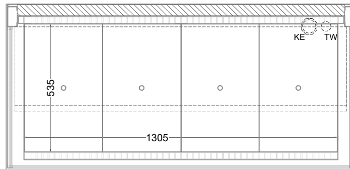
(Grundriss)
