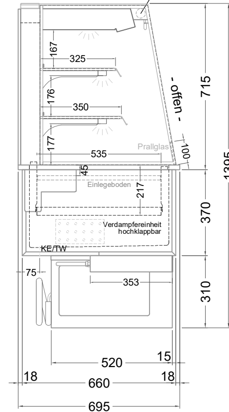
(Seitenansicht)
