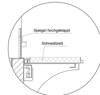
(Detail Spiegelsystem)
