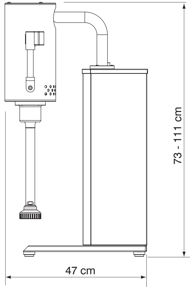
Seitenansicht
