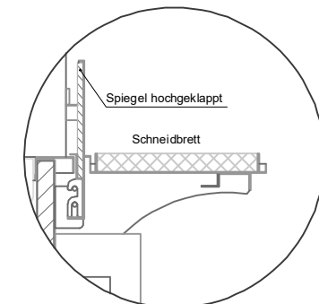
(Detail Spiegelsystem)
