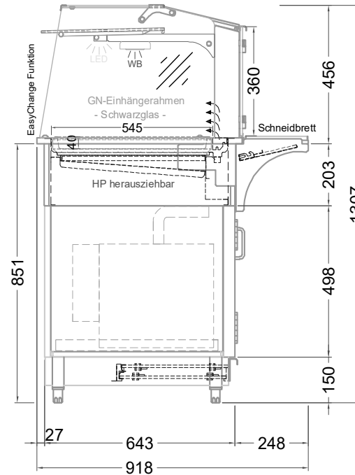
(Seitenansicht)
