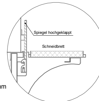
(Detail Spiegelsystem)
