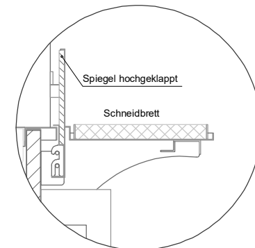
(Detail Spiegelsystem)
