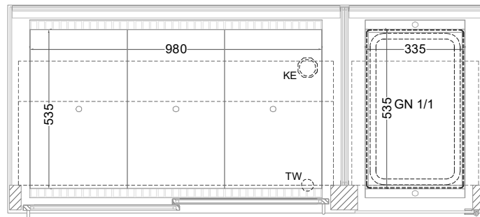
(Grundriss)
