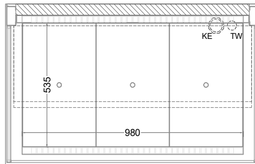
(Grundriss)
