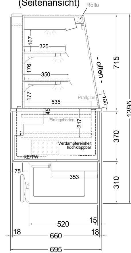
(Seitenansicht)
