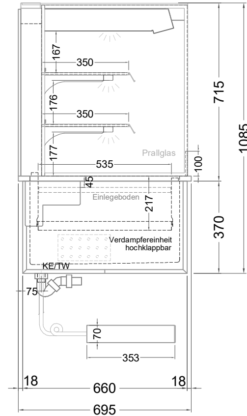
(Seitenansicht)
