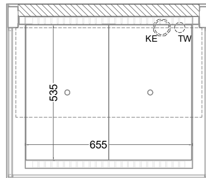
(Grundriss)
