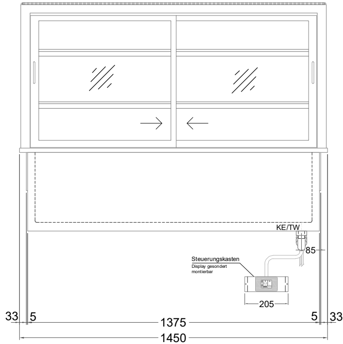
(Bedienseite)
