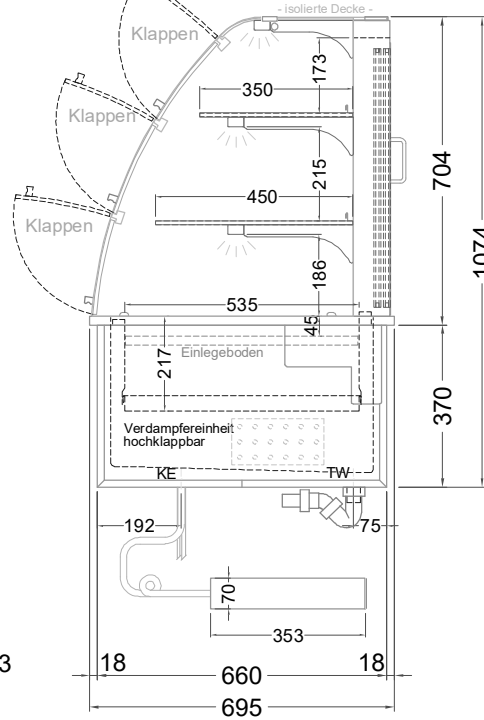
(Seitenansicht)
