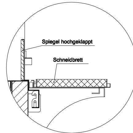
(Detail Spiegelsystem)
