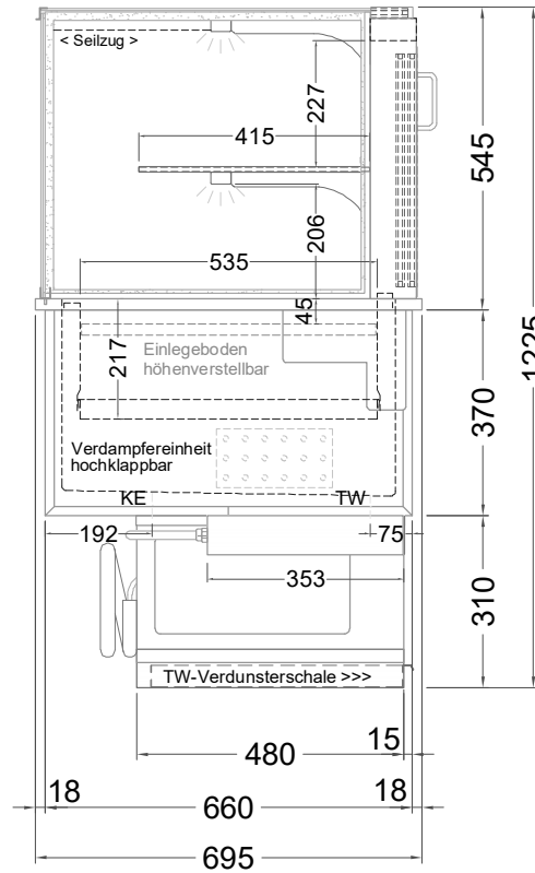
(Seitenansicht)
