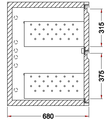
Schnitt L1
