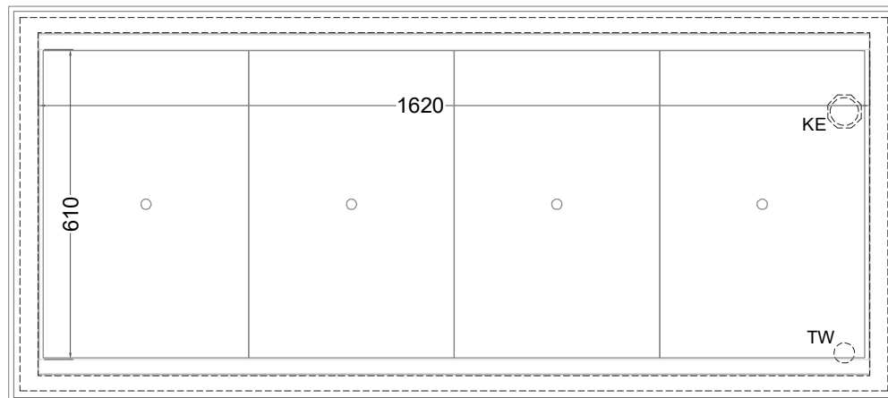
(Grundriss)
