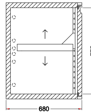
Schnitt Türelement
