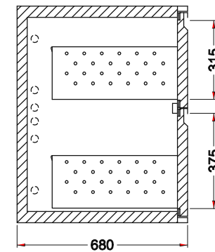
Schnitt L1
