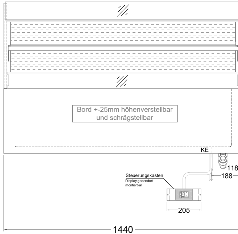
(Vorderseite)
