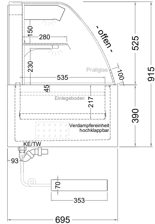
(Seitenansicht)
