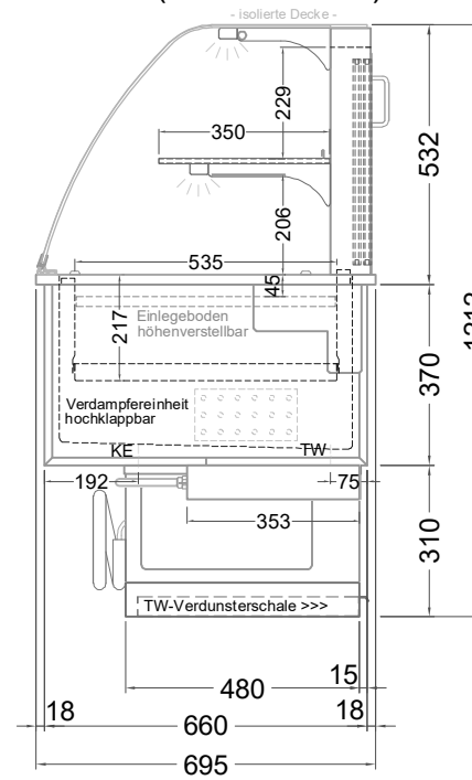
(Seitenansicht)
