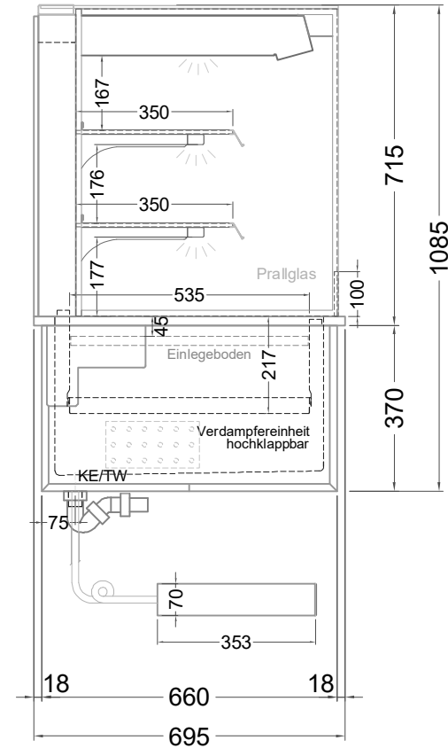
(Seitenansicht)
