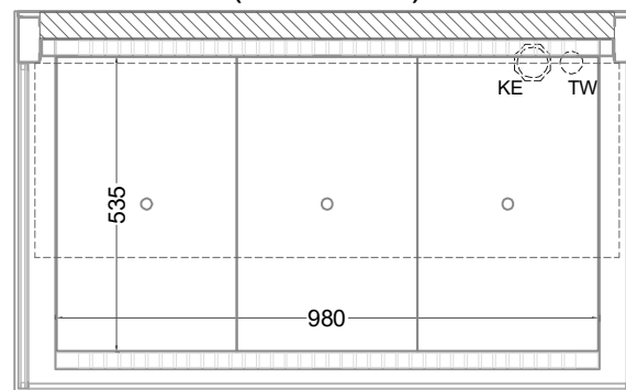
(Grundriss)
