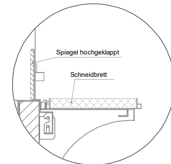
(Detail Spiegelsystem)
