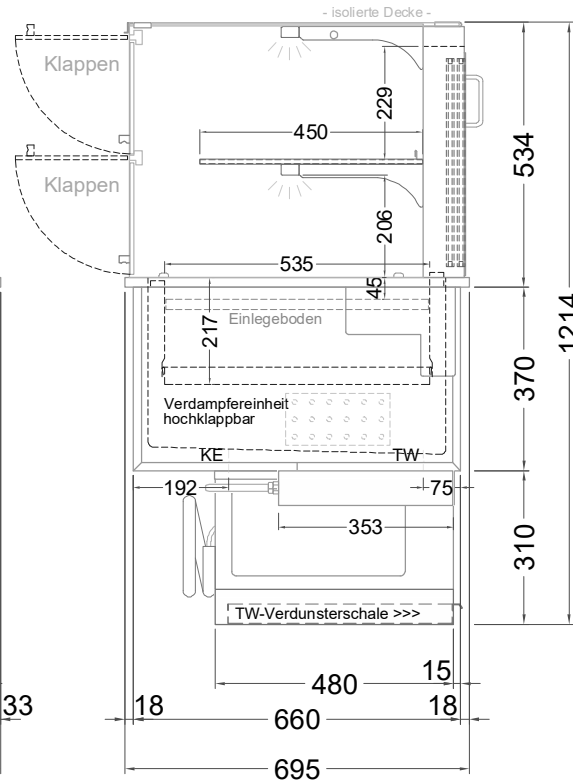
(Seitenansicht)
