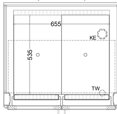
(Grundriss)
