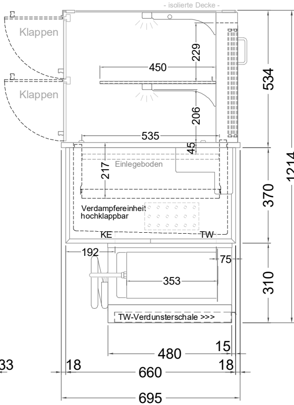
(Seitenansicht)
