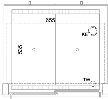
(Grundriss)
