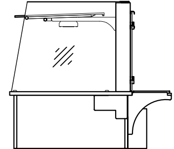
(Seitenansicht)
