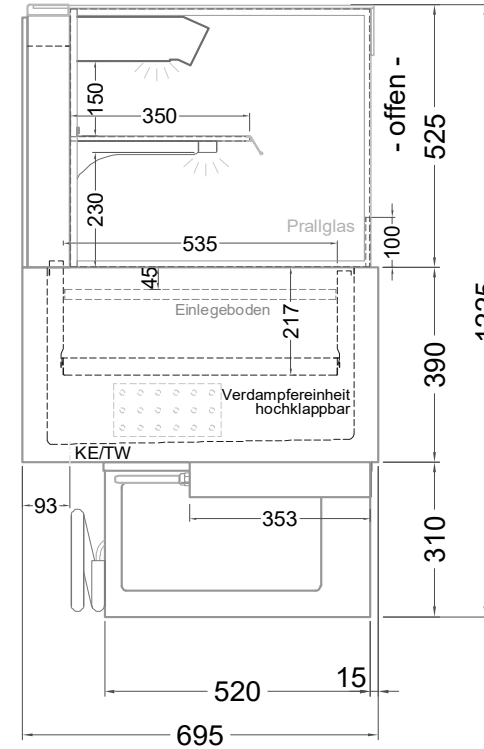
(Seitenansicht)
