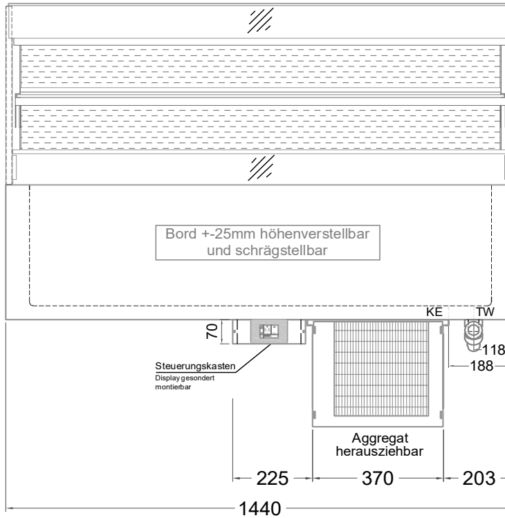
(Vorderseite)
