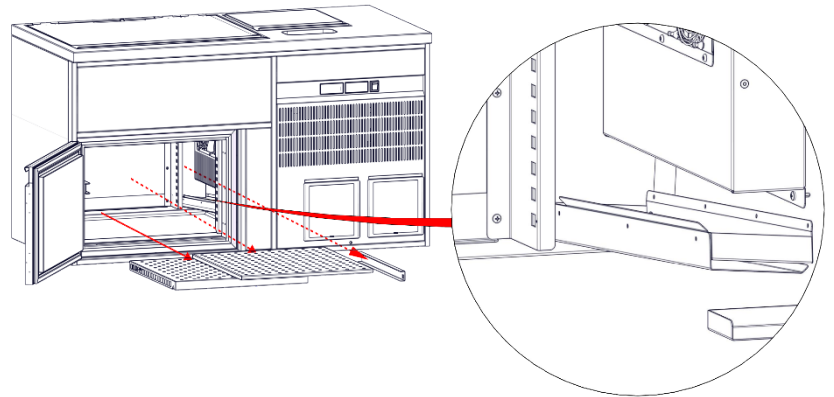
Abbildung 12: Tauwasserschale
