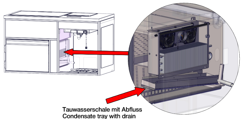
Abbildung 5: Tauwasseranschluss
