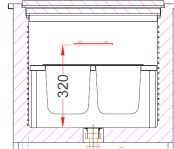
Abbildung 9: Stapelmarke Wanne
