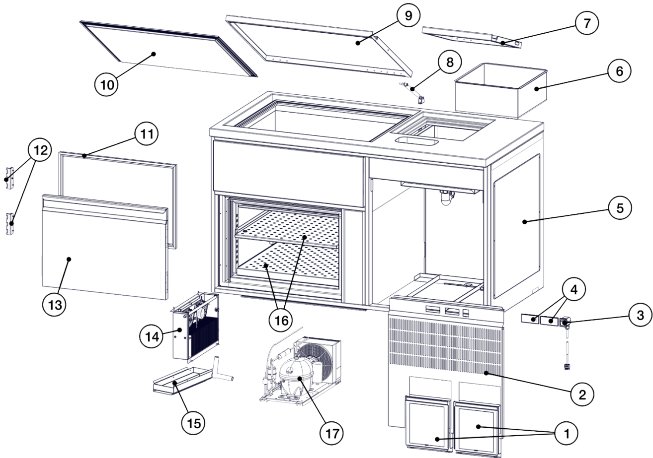
Abbildung 14: Teileübersicht
