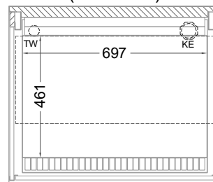
(Grundriss)
