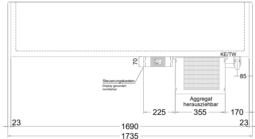
(Bedienseite)
