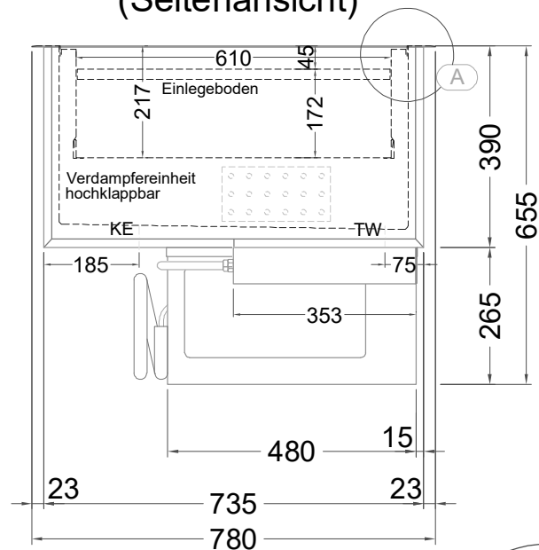
(Seitenansicht)
