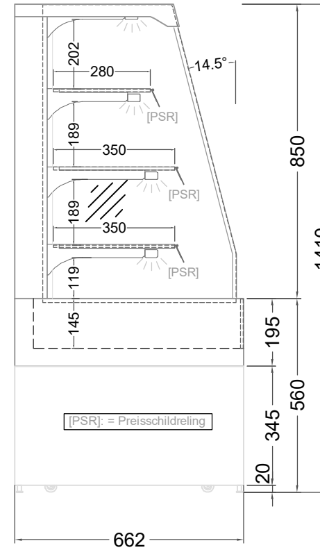
(Seitenansicht)
