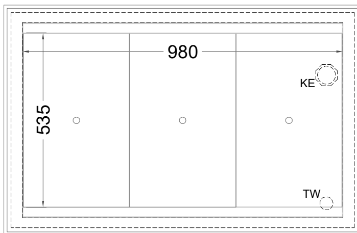
(Grundriss)
