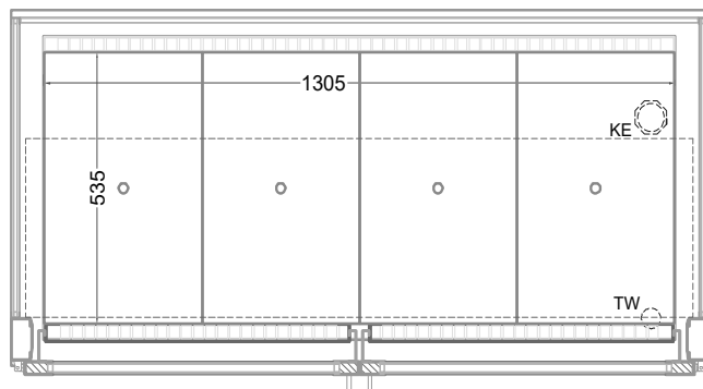
(Grundriss)
