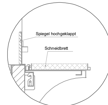
(Detail Spiegelsystem)
