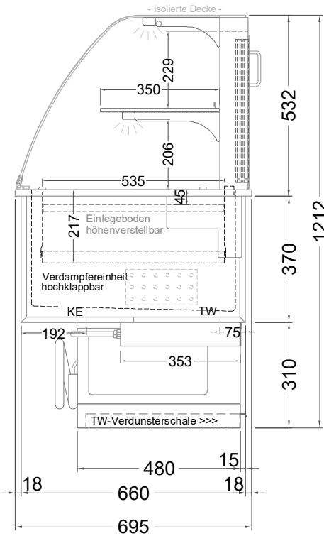
(Seitenansicht)
