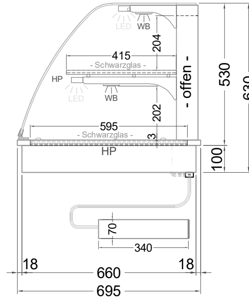
(Seitenansicht)
