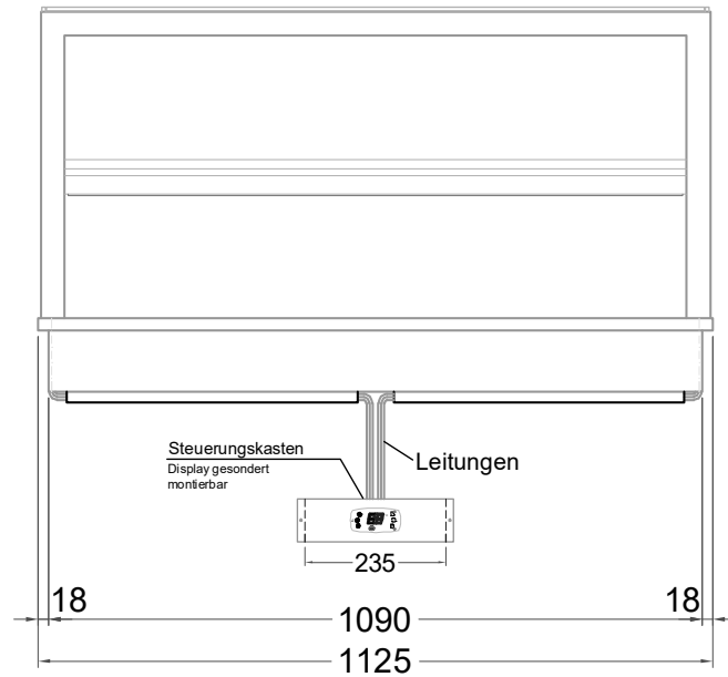
(Grundriss)
