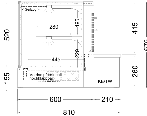
(Seitenansicht)
