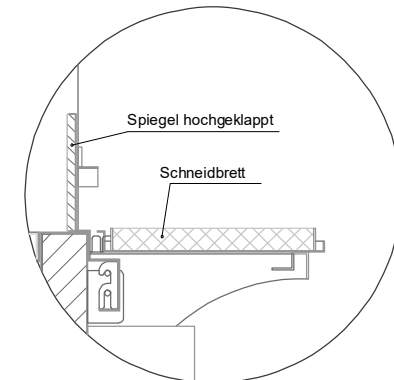
(Detail Spiegelsystem)
