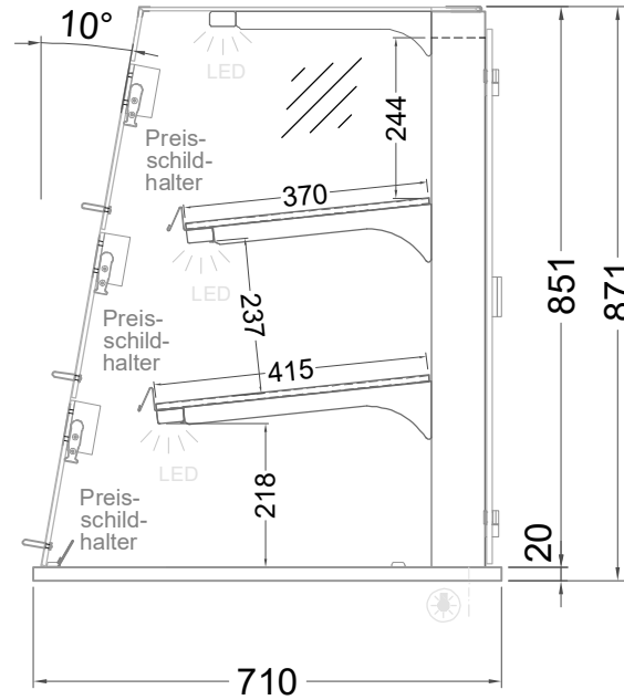
(Seitenansicht)
