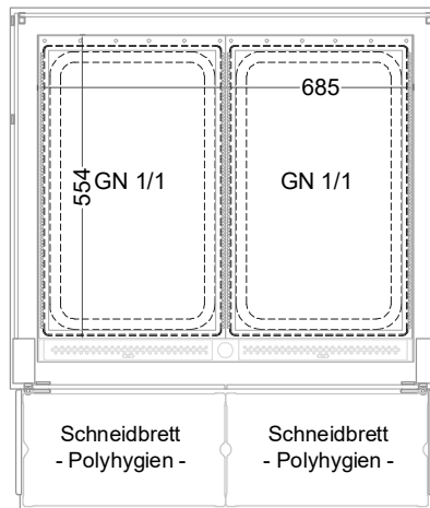
(Grundriss)
