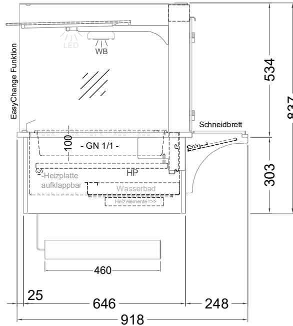
(Seitenansicht)
