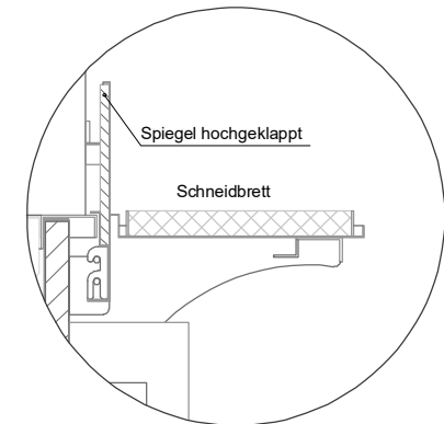
(Detail Spiegelsystem)
