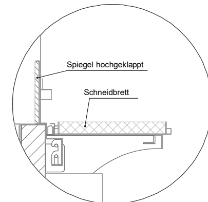
(Detail Spiegelsystem)
