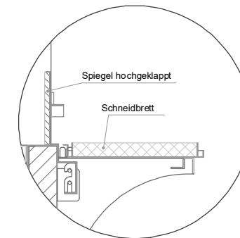
(Detail Spiegelsystem)
