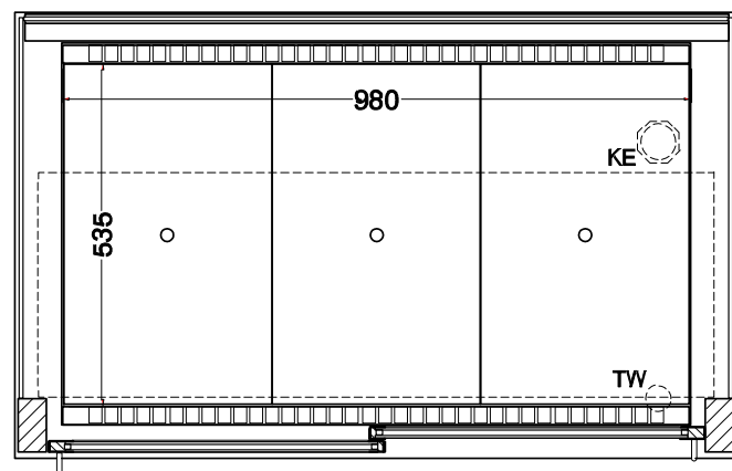
(Grundriss)
