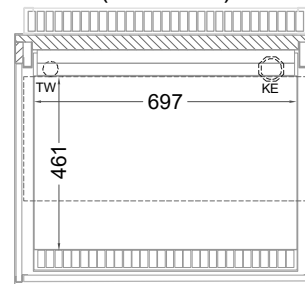
(Grundriss)
