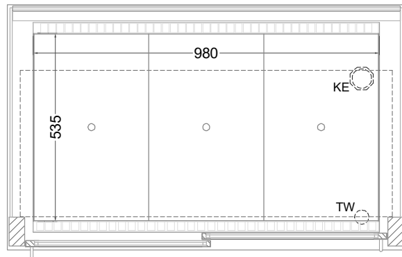
(Grundriss)
