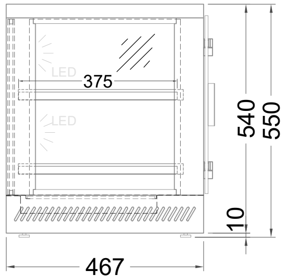
(Seitenansicht)
