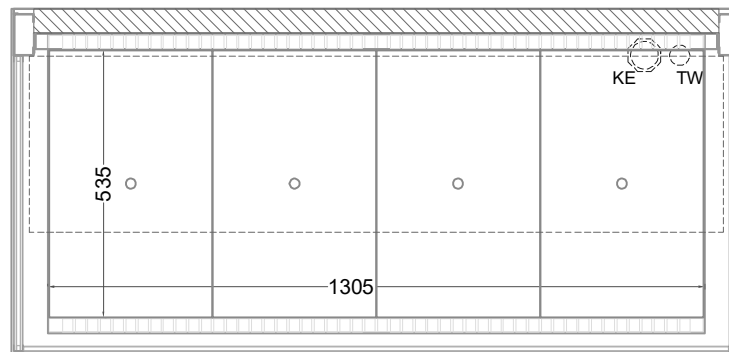
(Grundriss)
