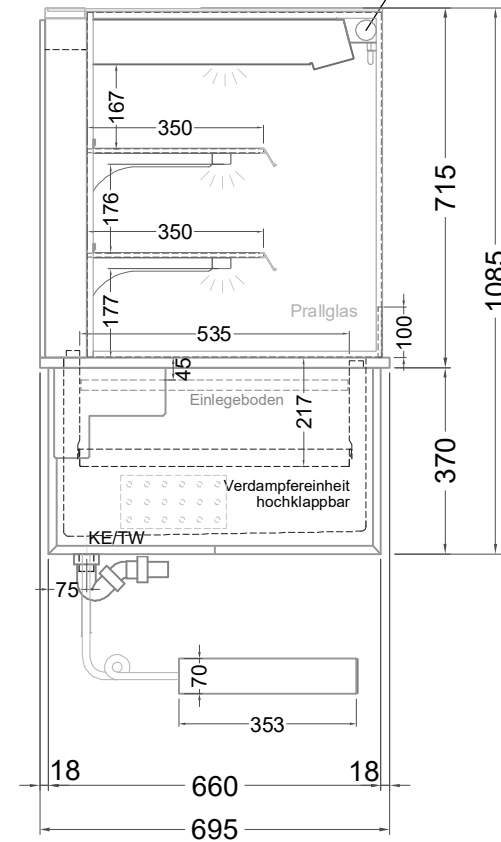
(Seitenansicht) Rollo
