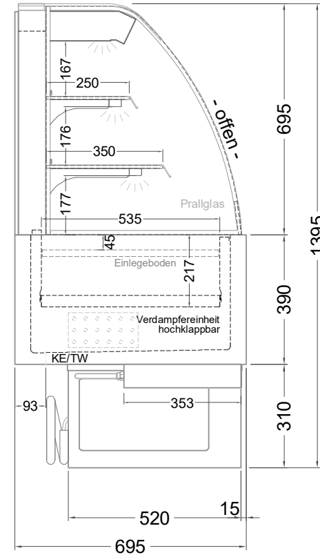
(Seitenansicht)
